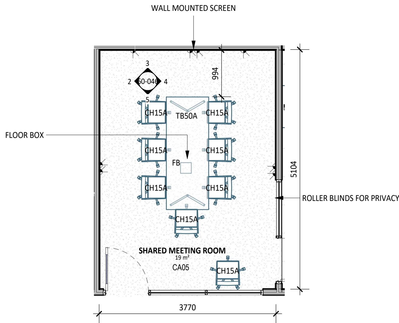
1 PLAN DETAIL 1 : 50
